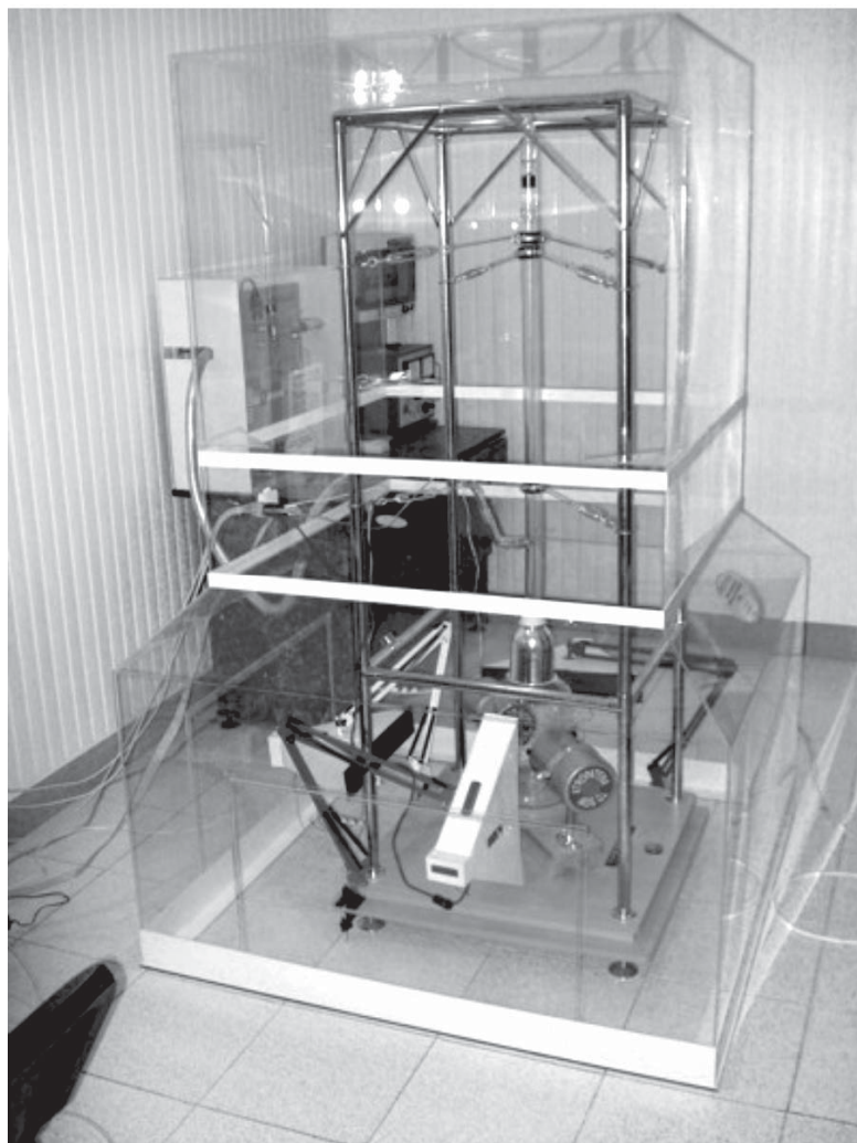
Рис. 53. Фотография Торсионного Детектора Длиннопериодных Гравитационных Вариаций (ТД ДГВ - АТРОПАТЕНА), расположенного на станции прогнозирования землетрясений НИИ прогнозирования и изучения землетрясений (г. Баку).
