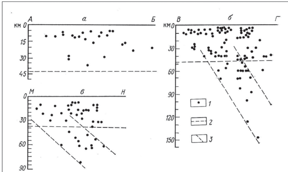
Рис.4, б. Профили через: а – Рионскую низменность; б – вкрест простирания восточной части Большого Кавказа; в – вкрест простирания Апшеронского порога на Каспии (Халилов Э.Н., Мехтиев Ш.Ф., Хаин В.Е., 1987).
