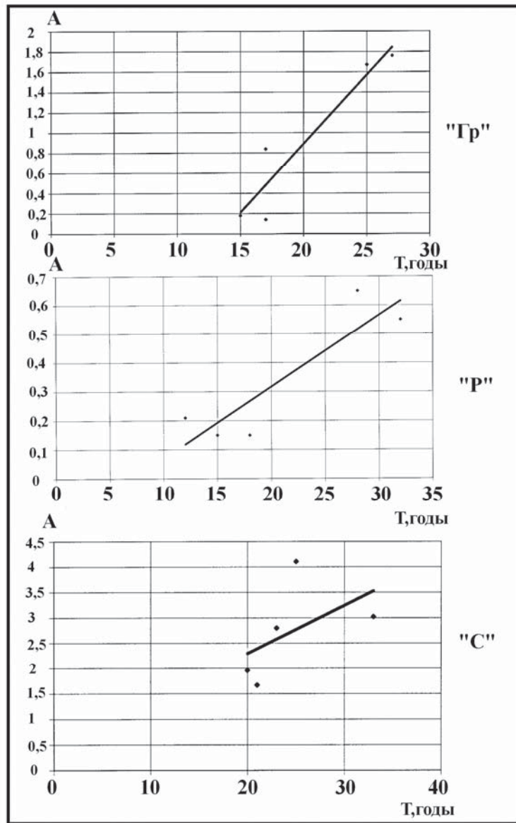
Рис.17. График зависимости периода между максимумами циклов вулканической активности T и относительной амплитудой последующего цикла активизации A для вулканов типов Gr, P и C.
