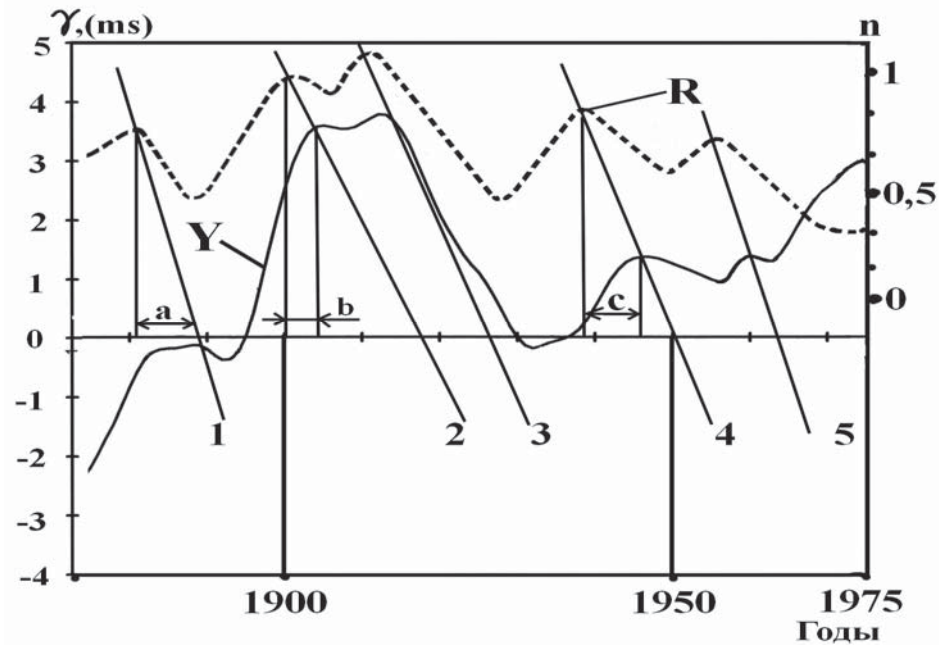
Рис.10. Фрагмент сопоставления графиков вариаций длительности земных суток и активности магматических вулканов типа R .
