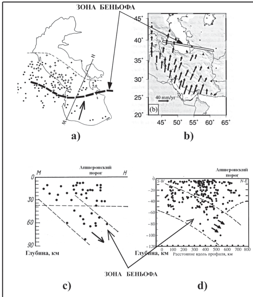
Рис.4 в. Схемы выявления зоны Беньюфа на Каспии различными авторами.
