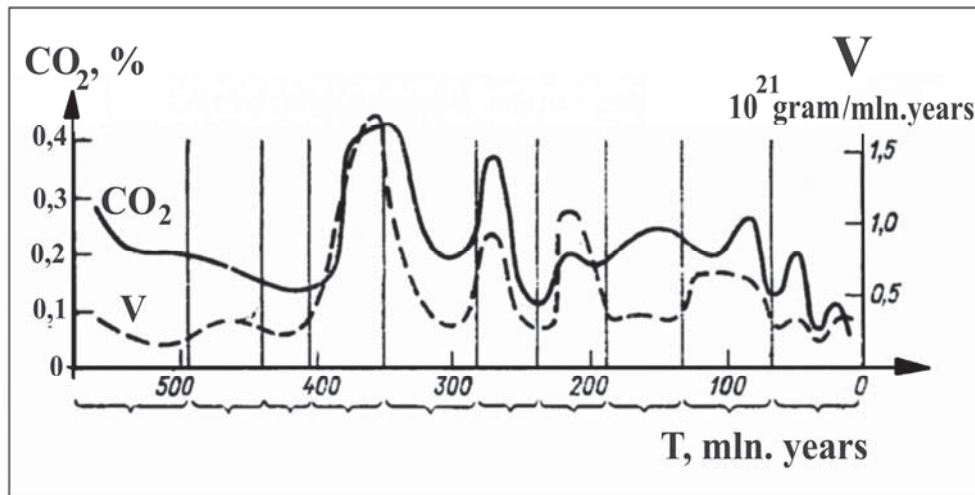
Рис.70. Изменения количества углекислого газа в атмосфере и скорость образования вулканогенных пород в течение фанерозоя (Athaturon M.L. and others, 1986).
